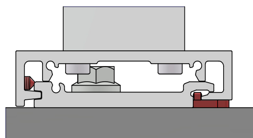
korrekt montierte Aushebelsicherung correctly fitted anti-lift device
