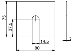
Ausgleichsblech für aufgesetzte Montage | shim plate for top mounting
