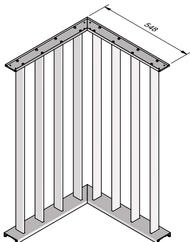
90° Außenecke | 90° external corner 1473R9005FS-AE1000
