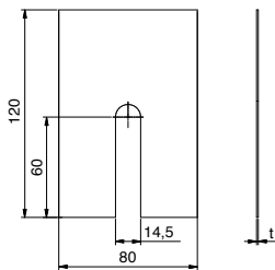
Ausgleichsblech für vorgesetzte Montage | shim plate for front mounting
