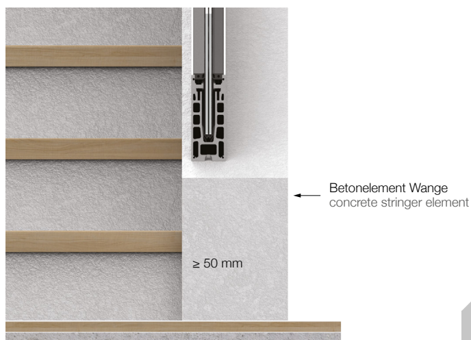
(E) Innenanwendung: Beispiel Treppe mit Betonelement Wange interior application: example staircase with concrete stringer element
