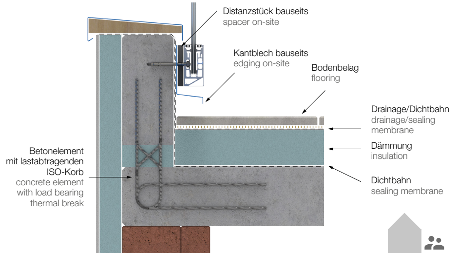
(C) Außenanwendung: Beispiel Balkon-Attika, gedämmt, Profil innen exterior application: example balcony attica, insulated, profile inside
