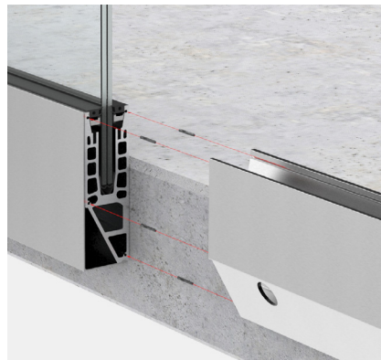
8. Verbinden von zwei Profilen mit Verbindungsstiften möglich connect two profiles with connector stud if necessary
