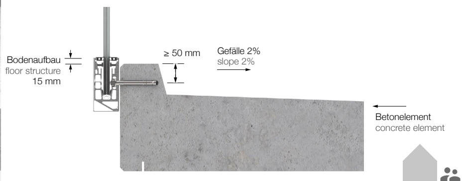
(B) Außenanwendung: Beispiel Balkon mit Betonelementen, Gefälle nach innen exterior application: example balcony with concrete elements, slope inwards
