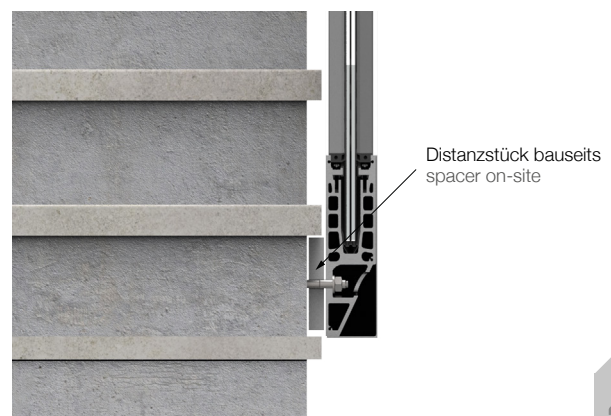
(E) Innenanwendung: Beispiel Treppe mit Überstandsstufen interior application: example staircase with overhang steps
