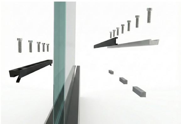
4. Druckleiste einsetzen | insert clamping bar links: PA6-Klemmleisten für VSG / PVB 1,52 mm left: PA6 clamp bar for VSG / PVB 1,52 mm rechts: Aluminium-Klemmleisten für VSG / PVB 0,76 mm right: aluminium clamp bar for VSG / PVB 0,76 mm
