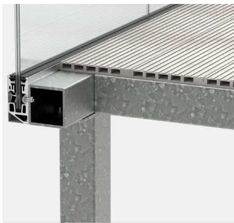
(A) Außenanwendung: Beispiel vorgesetzter Anbaubalkon exterior application: example front mounted balcony
