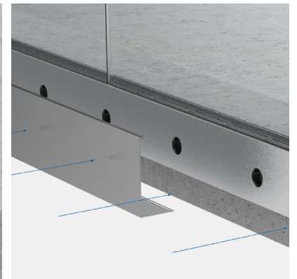
6. Blende einsetzen. insert the cladding.
