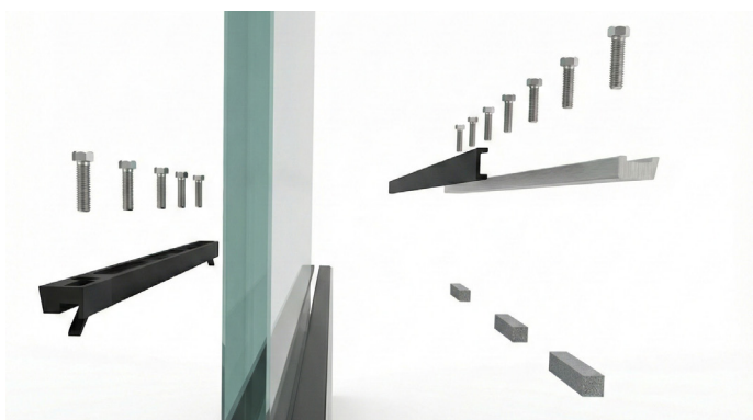
4. Druckleiste einsetzen | insert clamping bar links: PA6-Klemmleisten für VSG / PVB 1,52 mm left: PA6 clamp bar for VSG / PVB 1,52 mm rechts: Aluminium-Klemmleisten für VSG / PVB 0,76 mm right: aluminium clamp bar for VSG / PVB 0,76 mm
