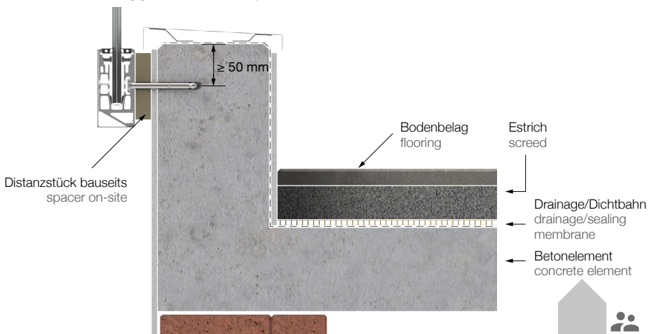
(D) Außenanwendung: Beispiel Balkon-Attika, Profil außen exterior application: example Balkon-Attika, Profil außen
